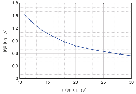
PAX1直行程执行器电流消耗特征曲线
