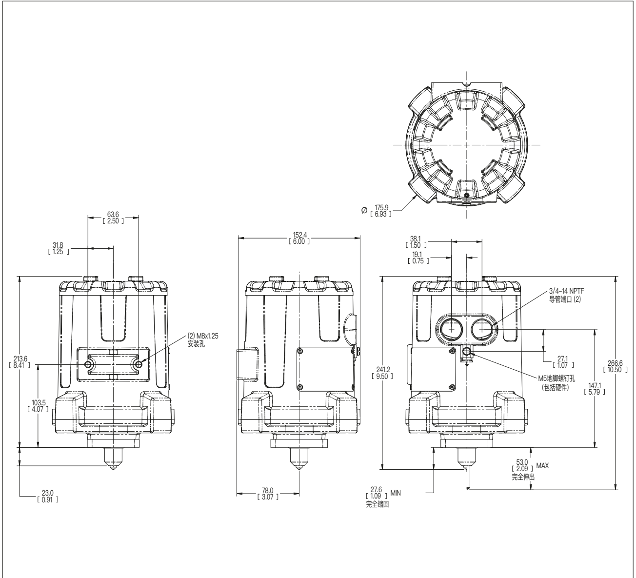
图 13 PAX1执行器
