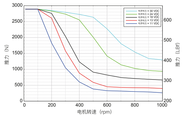
PAX1执行器 推力与电机转速和电源电压的关系
