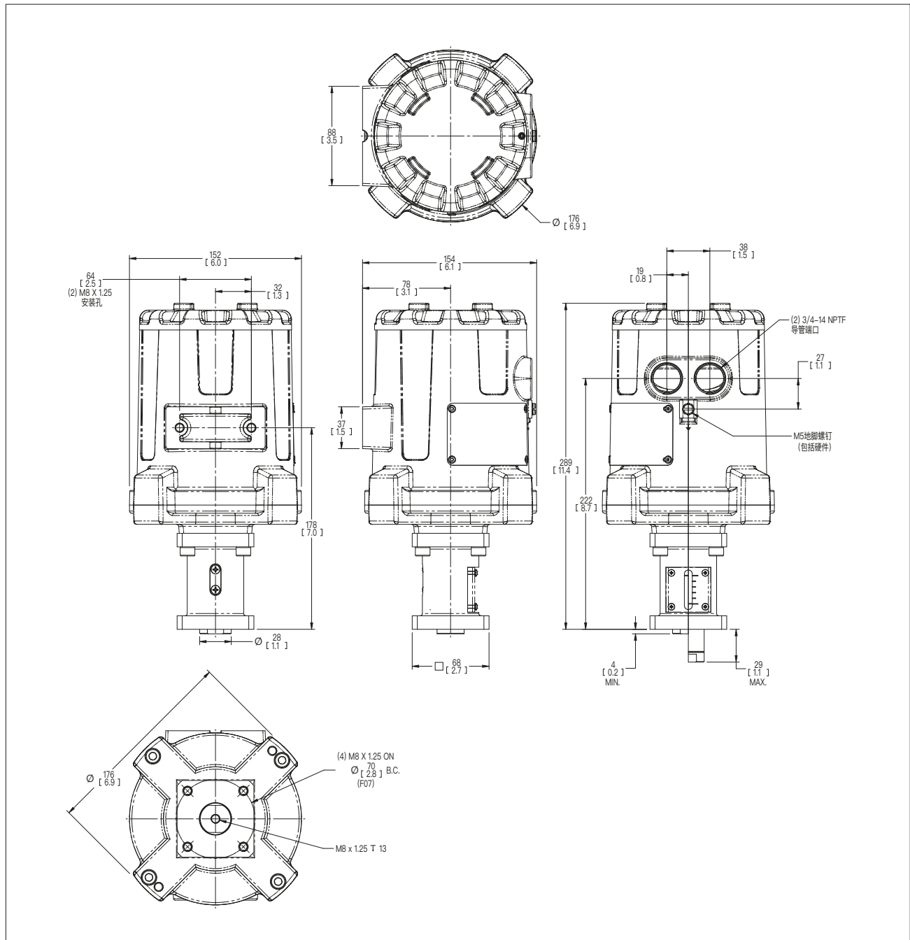
图 14 PAXL 执行器
