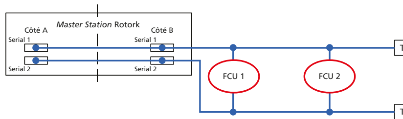
Fig 8.1.5: Topologie à deux canaux
