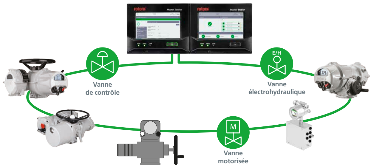
Fig 8.1: Anneau redondant ouvert Modbus
