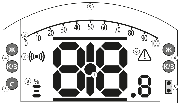
Рис. 6.4.1. Сегментный дисплей
