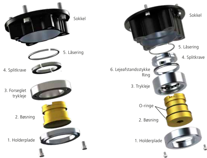
Fig. 5.1.2 F10-sokkelsamling
