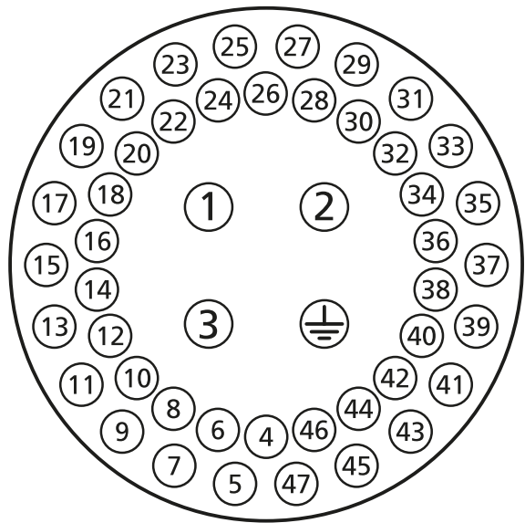
图. 7.1.1 接线端子的接线需参考执行器的电气接线图
